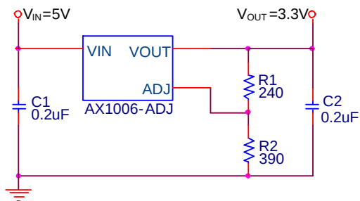
ADJ Output
