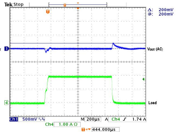
Load Transient ( V_{IN}=12V , V_{OUT}=2.5V , Load=0~2A)
