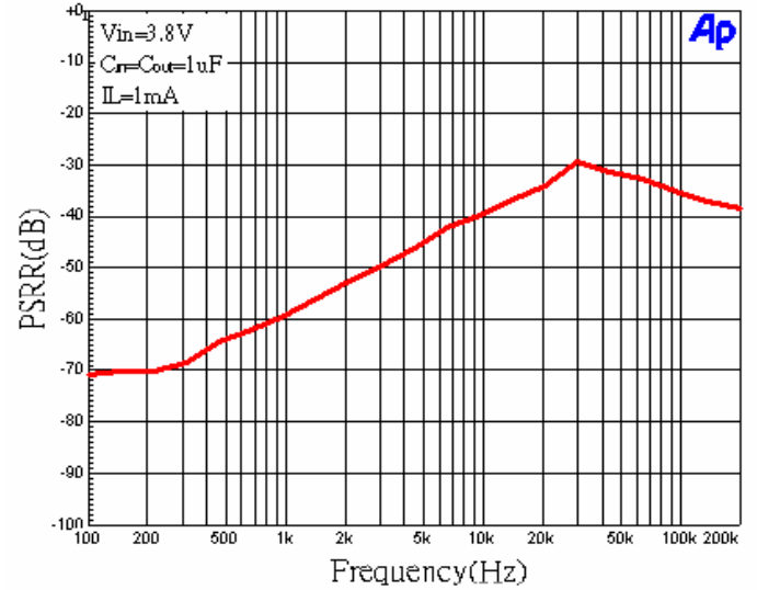
PSRR
