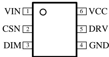
SOT23-6
