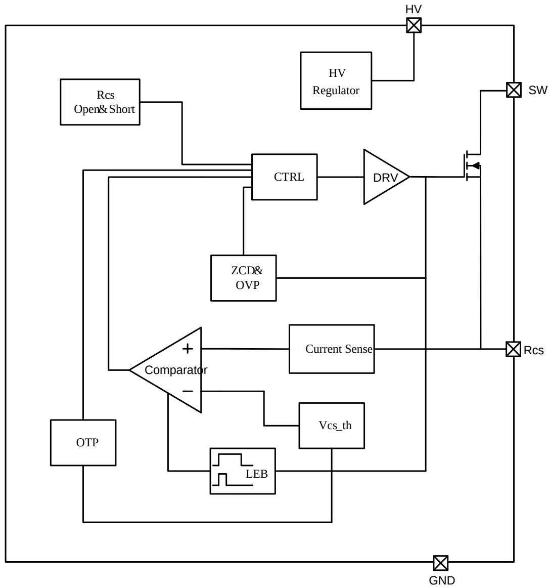
简化模块图
