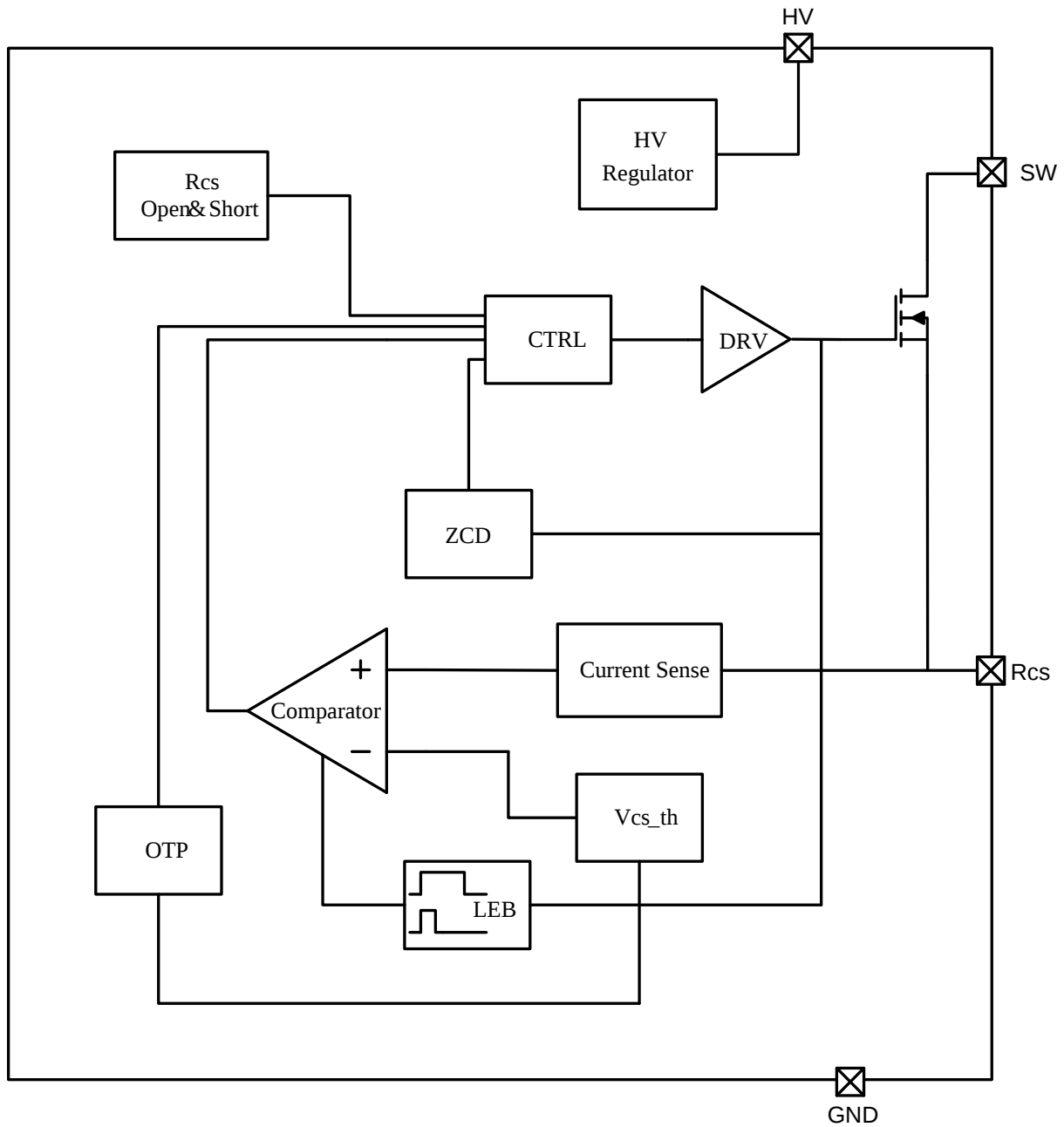
简化模块图
