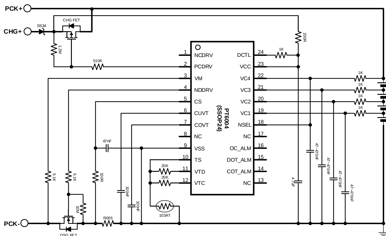
图 2. 充电 PMOSFET 和放电 NMOSFET 的典型 4 串电池包应用电路
