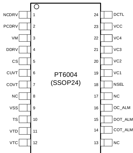
图 7. 管脚定义图
